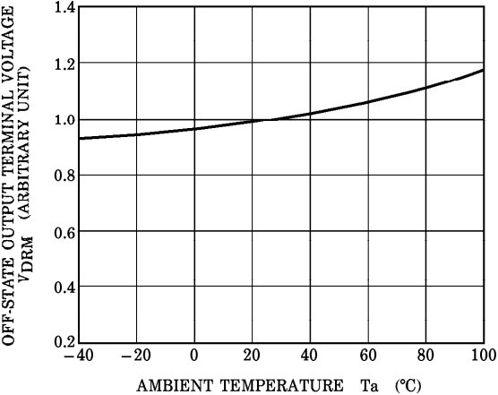
NORMALIZED V_{DRM} - T_a
