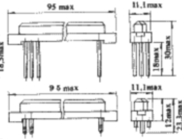
Розетка СИИ59 Socket
