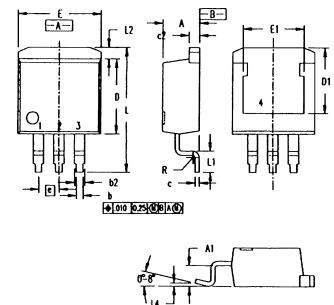
TO-263 AA Outline
