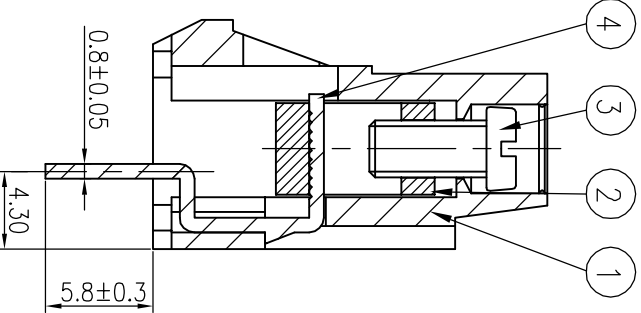
截面 A-A
