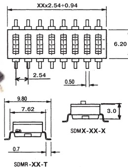
DIP ВДМ-1-xx (угловой)
