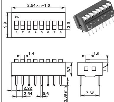
DIP ВДМ-1-xx (угловой)
