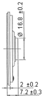
Dimension : Millimetres
