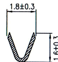
A-A SECTION
